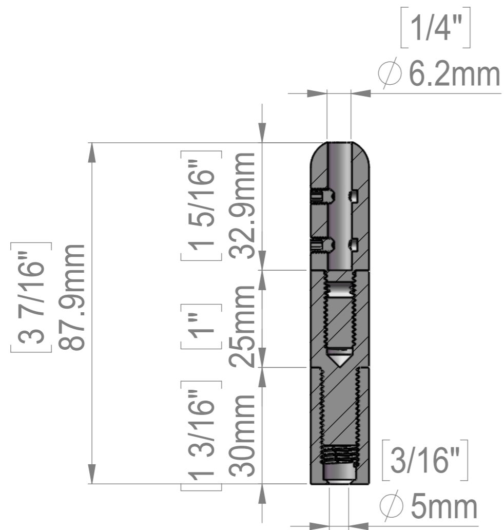
SECTION A-A
